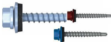
Sestorokutni vijak sa EPDM podloskom sa siljkom u boji 8117F11, csomagolás 250 db/doboz
